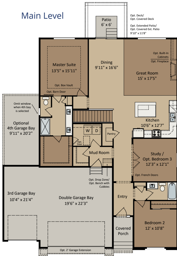
Optional Bedroom 3 in Lieu of Study
